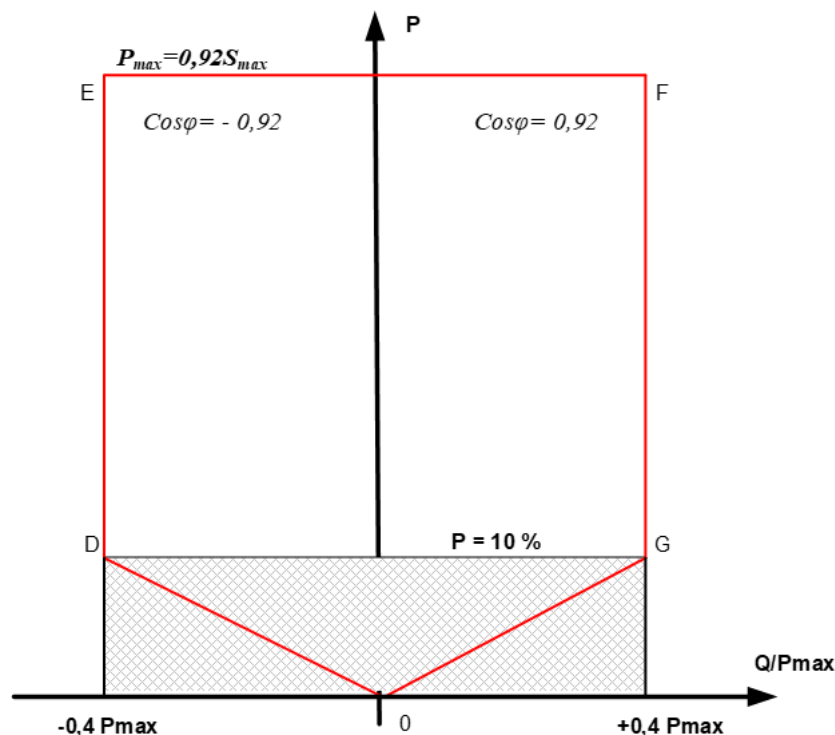
3 pav. D tipo EJP P-Q/Pmax charakteristikos profilis
